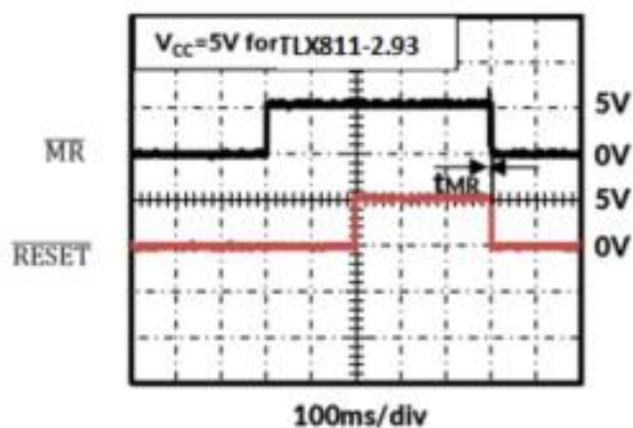
图 11. 复位时序
