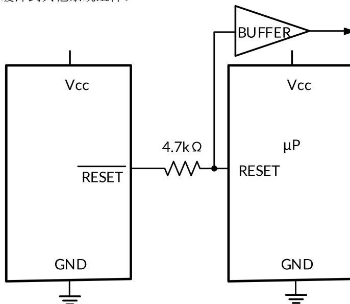
图 14. 缓冲 RESET 到其他系统组件
