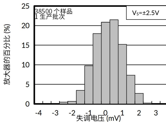
图 14. 失调电压分布
