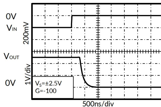
图 12. 正向过压恢复
