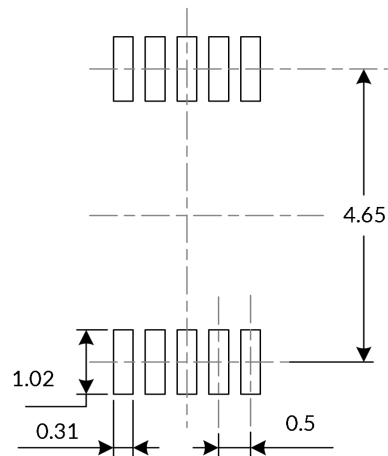
推荐焊盘尺寸 (单位: 毫米)
