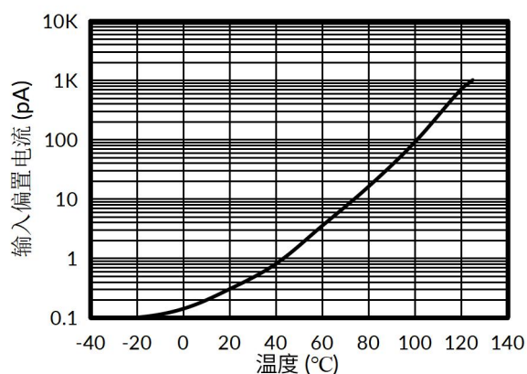
图 9. 输入偏置电流与温度的关系
