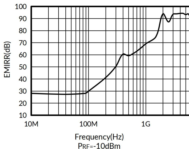
图 16. TLX82X EMIRR和频率的关系
