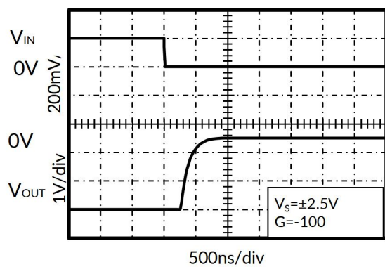
图 13. 反向过压恢复
