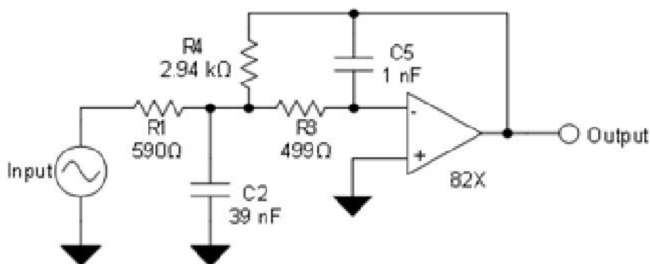
图 18. 25-kHz 低通滤波器
