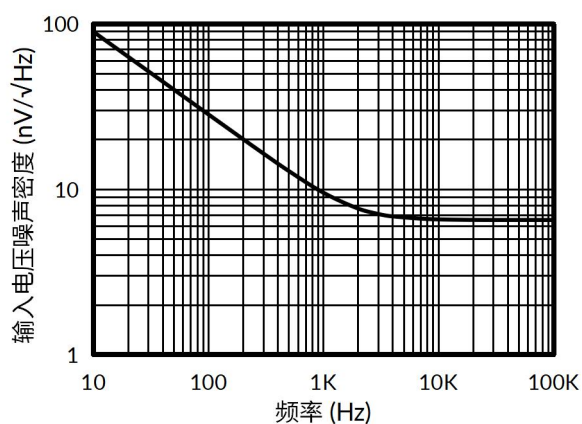
图 3. 输入电压噪声密度与频率的关系
