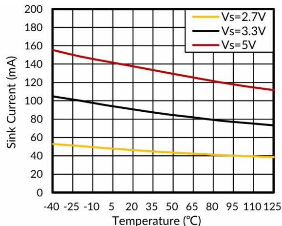
图 5. 灌电流与温度的关系
