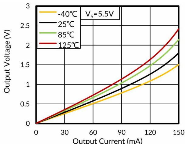
图 7. 输出电压摆幅与输出电流（灌电流）的关系
