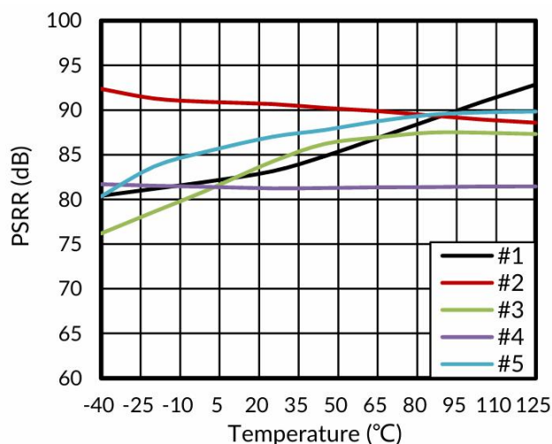
图 9. 电源抑制比与温度的关系
