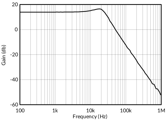
图 20. 低通滤波器
