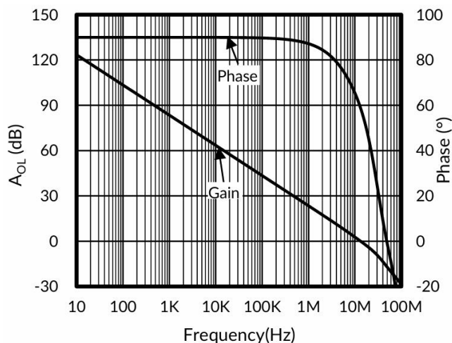
图 17. 开环增益和相位裕度与频率的关系
