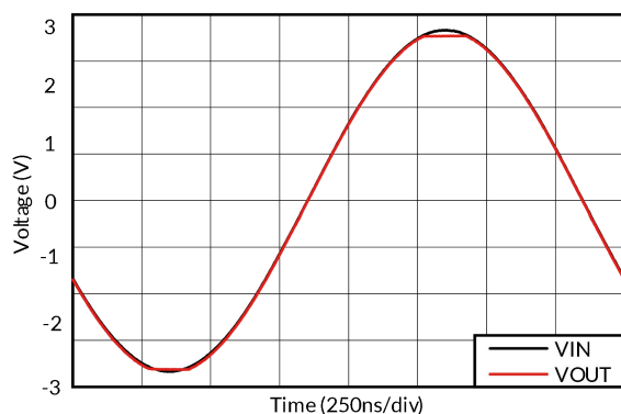
图 18. 在输入过驱动状态下无相位翻转的输出波形
