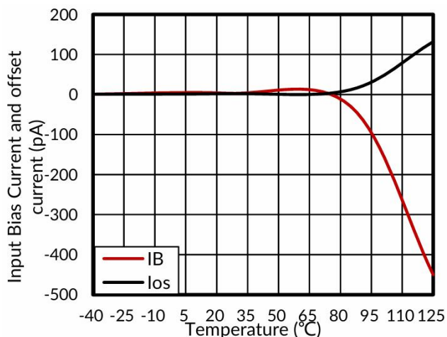
图 11. 输入偏置电流和失调电流与温度的关系
