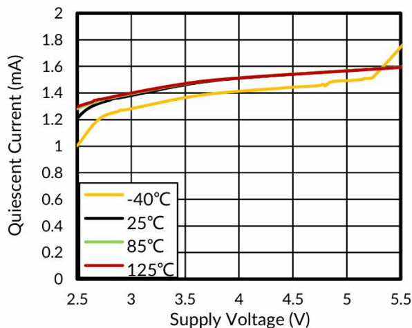
图 2. 静态电流与电源电压的关系
