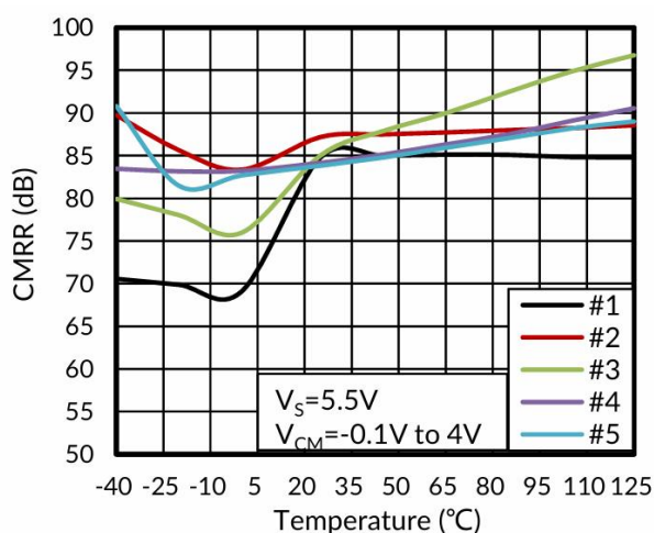
图 10. 共模抑制比与温度的关系
