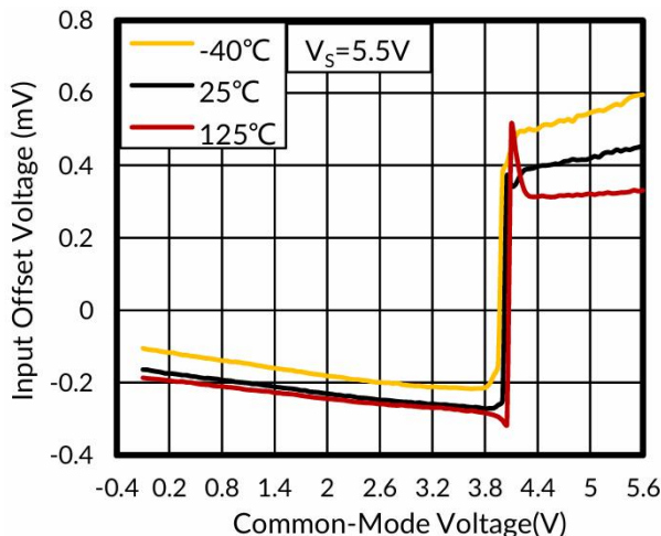
图 4. 输入失调电压与共模电压的关系
