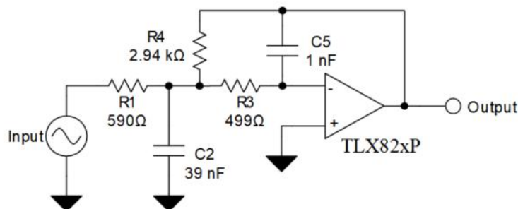
图 19. 25-kHz 低通滤波器
