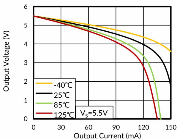
图 8. 输出电压摆幅与输出电流（拉电流）的关系
