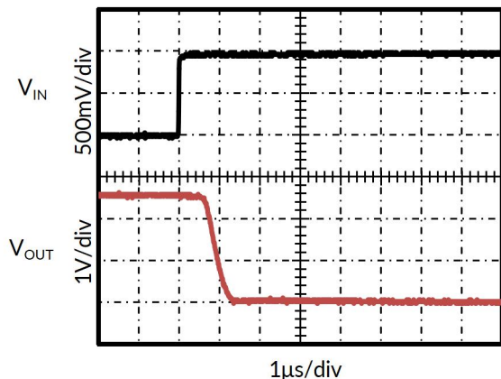
图 13. 正向过载恢复
