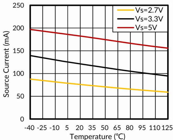
图 6. 拉电流与温度的关系
