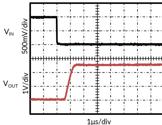
图 14. 反向过载恢复
