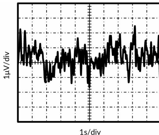
图 12. 0.1Hz ~ 10Hz 输入电压噪声
