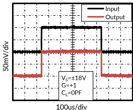
图 5. 小信号阶跃响应
