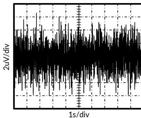
图 10. 0.1Hz~10Hz 输入电压噪声 AT V_S = 5\text{V}
