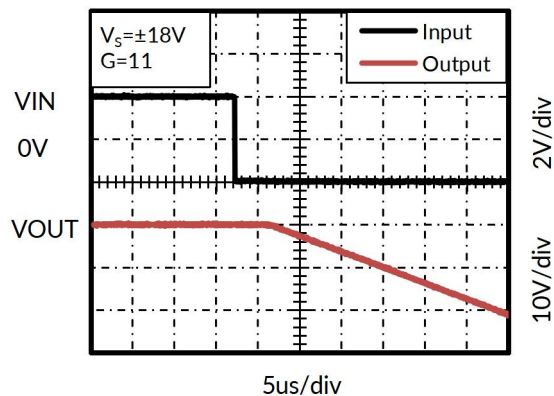
图 8. 反向过载恢复
