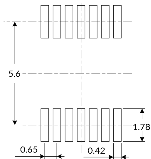
推荐焊盘尺寸 (单位: 毫米)
