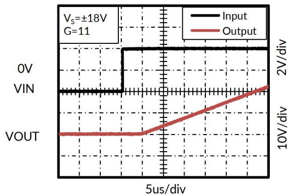
图 7. 正向过载恢复
