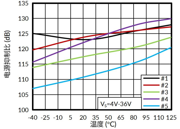
图 14. 电源抑制比与温度的关系
