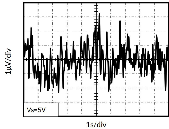
图 22. 0.1Hz~10Hz输入电压噪声
