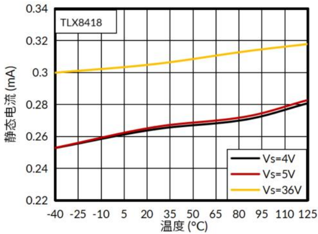
图 21. 静态电流与温度的关系
