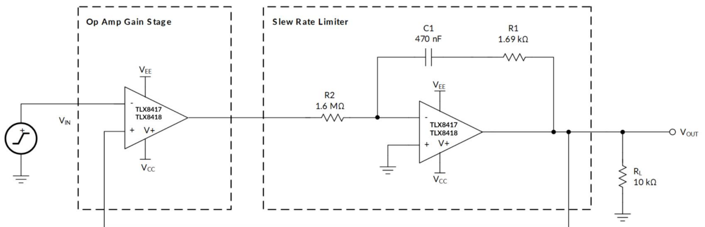
图 33. 压摆率限制器使用一个运算放大器
