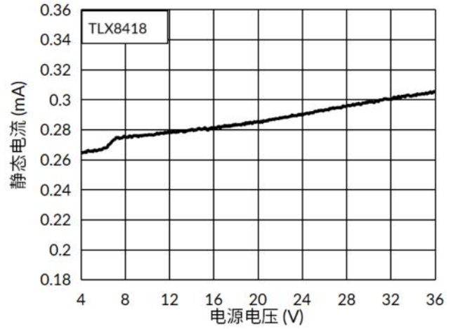
图 20. 静态电流与电源电压的关系
