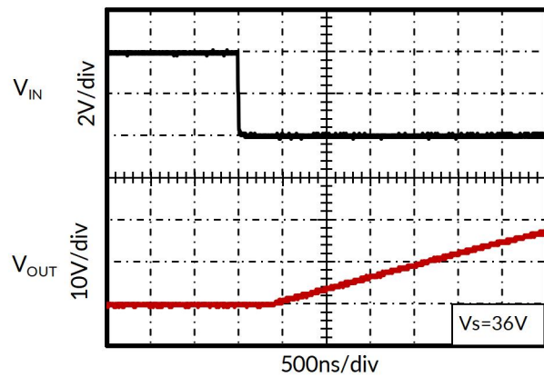
图 24. 反向过载恢复
