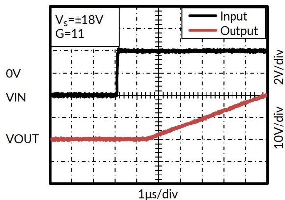
图 7. 正向过载恢复
