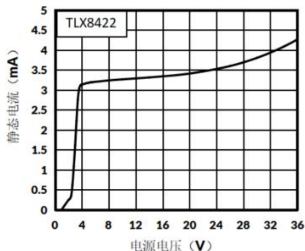
图 2. 静态电流与电源电压的关系
