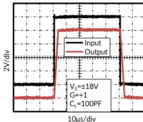
图 4. 大信号阶跃响应
