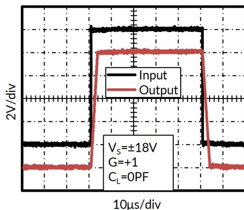
图 3. 大信号阶跃响应
