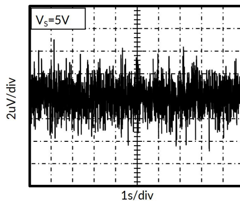
图 10. 0.1Hz~10Hz 输入电压噪声
