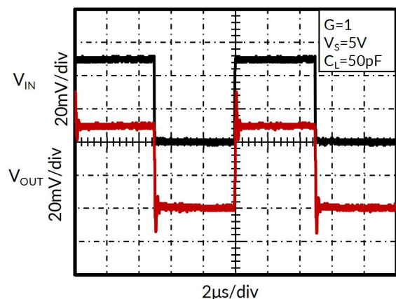
图 25. 小信号阶跃响应
