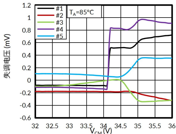
图 8. 失调电压与共模电压的关系 (切换区域)
