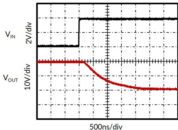
图 23. 正向过载恢复
