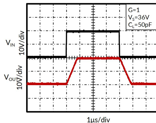
图 26. 大信号阶跃响应
