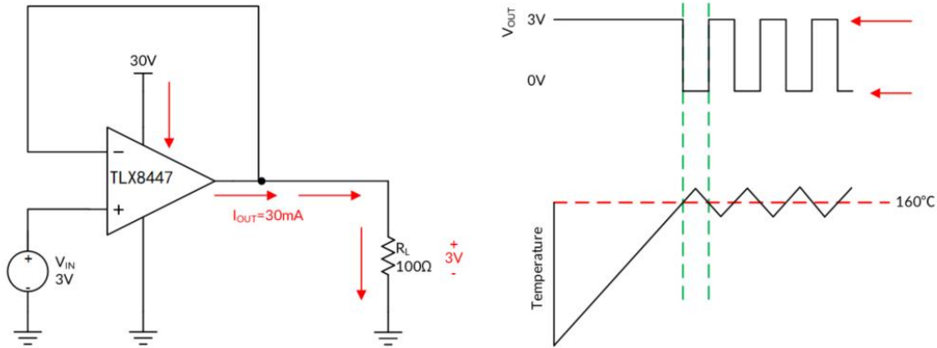
图 30. 过热保护
