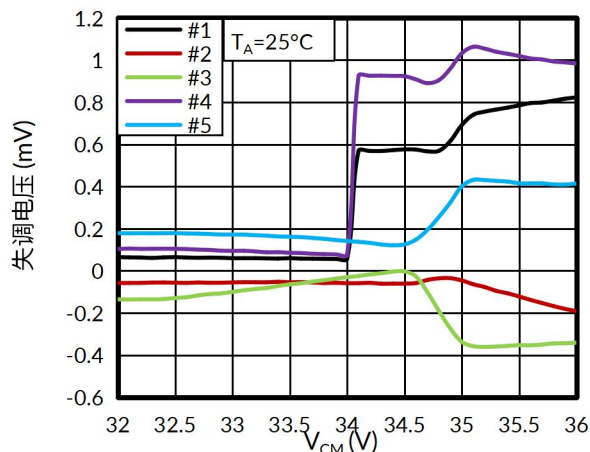
图 6. 失调电压与共模电压的关系 (切换区域)
