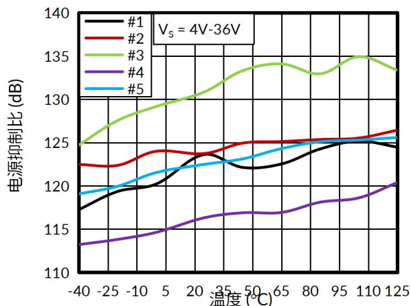
图 14. 电源抑制比与温度的关系
