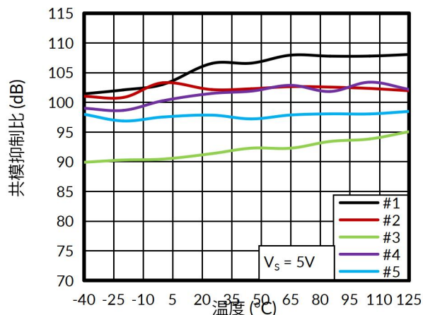
图 13. 共模抑制比与温度的关系
