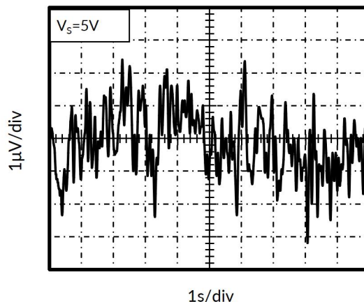
图 22. 0.1Hz~10Hz 输入电压噪声
