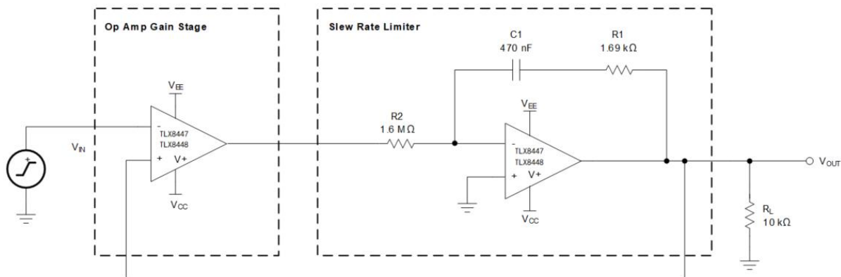
图 33. 压摆率限制器使用一个运算放大器
