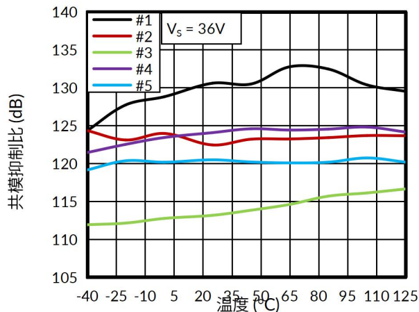
图 12. 共模抑制比与温度的关系
