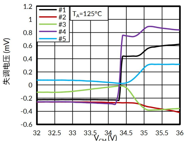
图 10. 失调电压与共模电压的关系 (切换区域)
