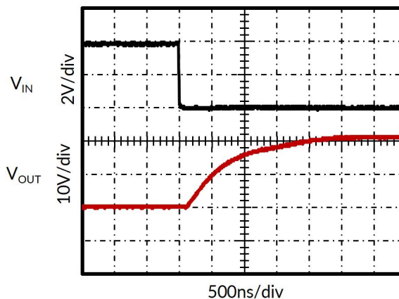
图 24. 反向过载恢复
