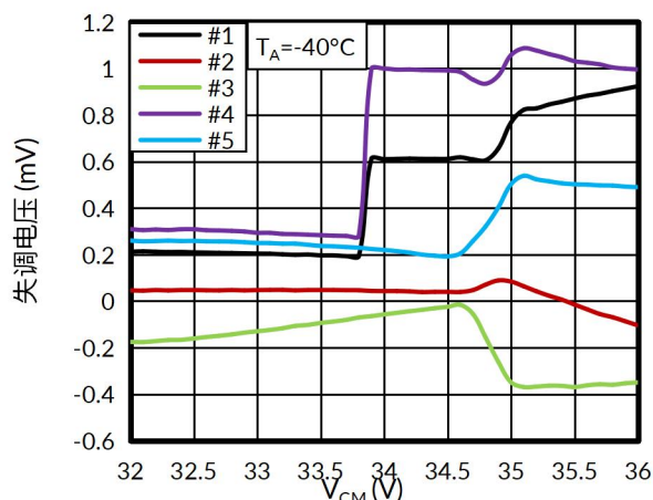
图 4. 失调电压与共模电压的关系 (切换区域)
