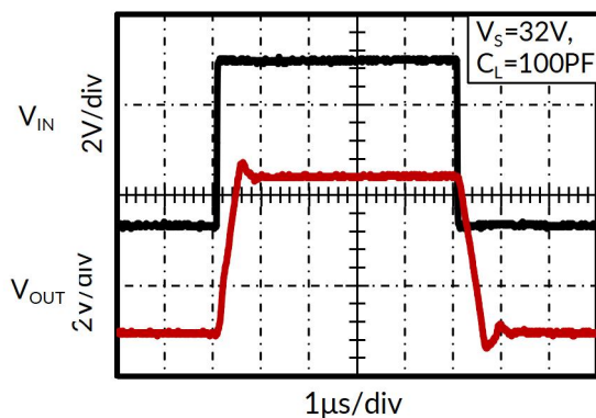
图 5. 大信号阶跃响应
