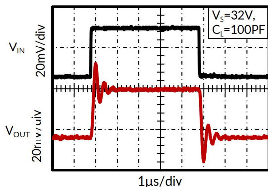
图 3. 小信号阶跃响应
