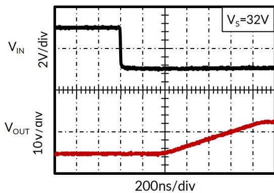
图 9. 反向过载恢复
