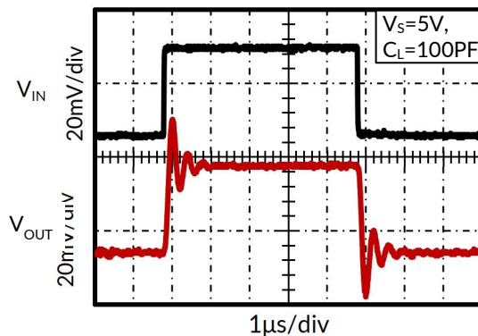
图 2. 小信号阶跃响应
