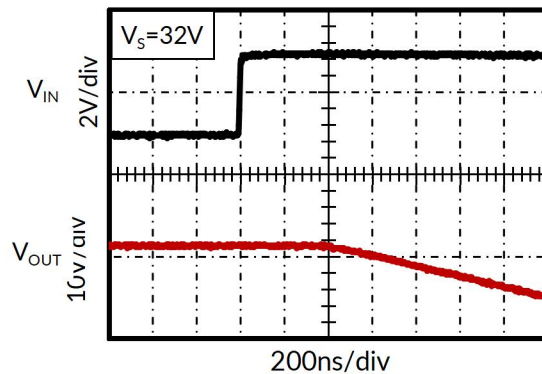
图 8. 正向过载恢复
