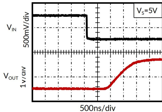
图 7. 反向过载恢复
