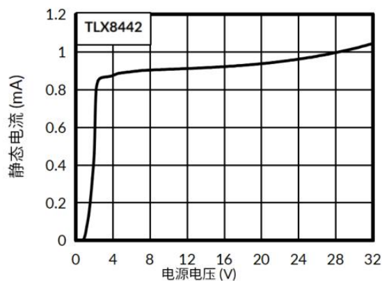
图 1. 静态电流与电源电压的关系
