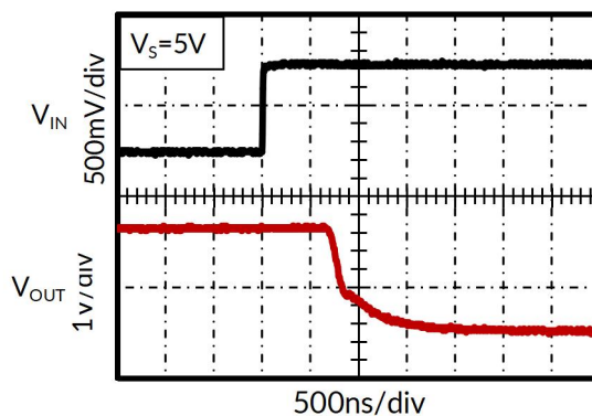
图 6. 正向过载恢复
