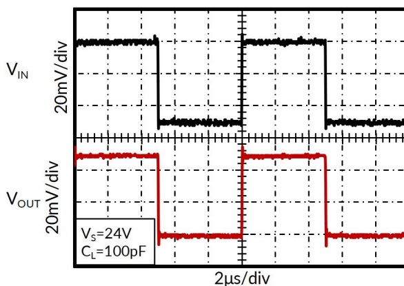
图 18. 小信号阶跃响应
