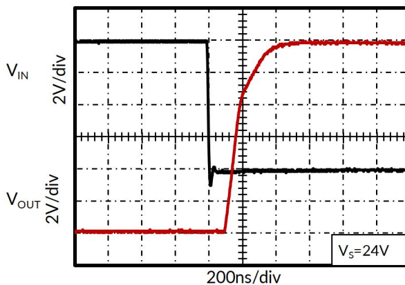
图 22.负过载恢复
