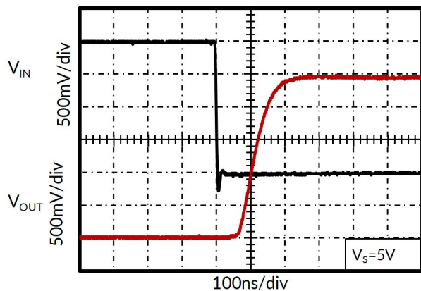
图 21.负过载恢复
