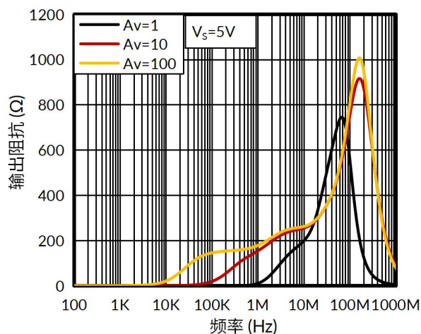
图 10. 输出阻抗与频率的关系
