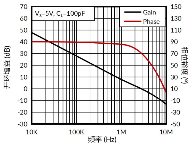
图 8. 开环增益和相位裕度与频率的关系
