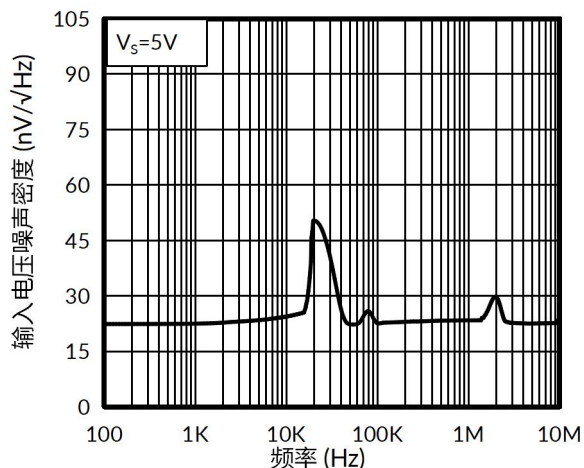
图 11. 输入电压噪声密度与频率的关系
