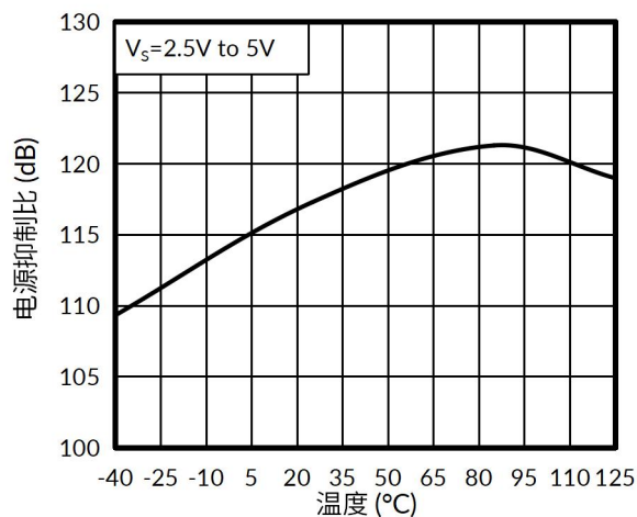
图 14. 电源抑制比与温度的关系
