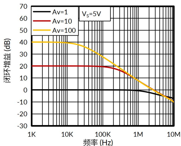
图 9. 闭环增益与频率的关系
