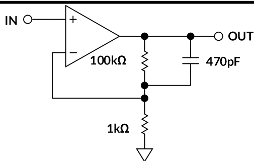
图 25. 一阶低通滤波器测试电路， \times 101 倍增益和 3kHz 截止频率
