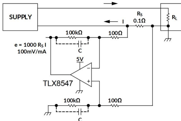
图 36. 低侧电流检测
