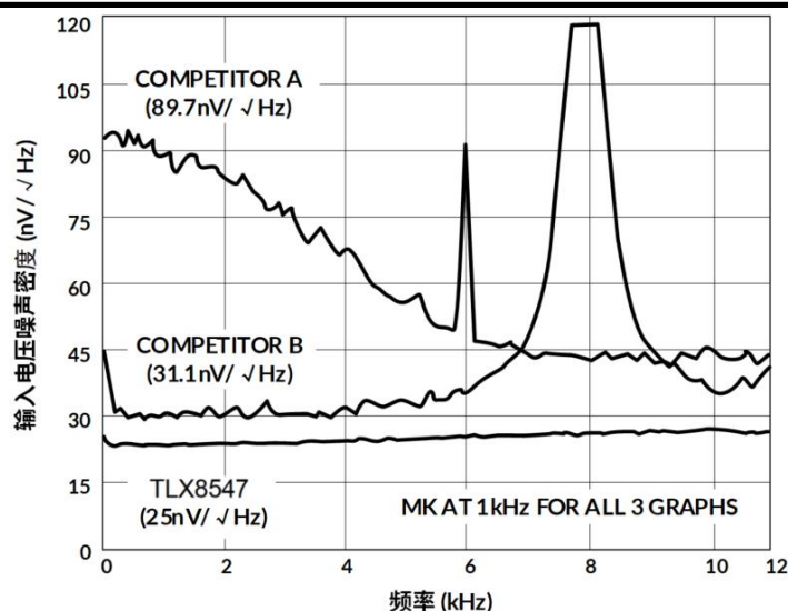
图 22. TLX8547 与竞品噪声频谱密度对比
