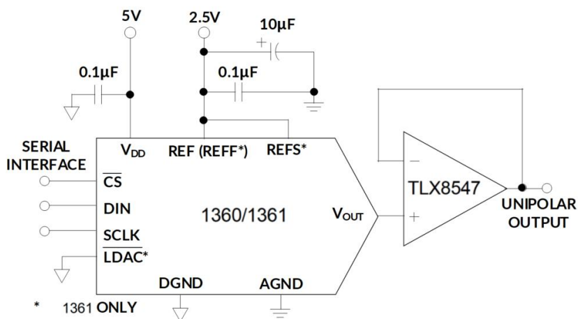
图 37. TLX8547 作为输出放大器应用方案
