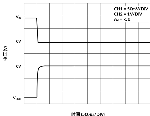
图 29. TLX8547 的正向输入过载恢复
