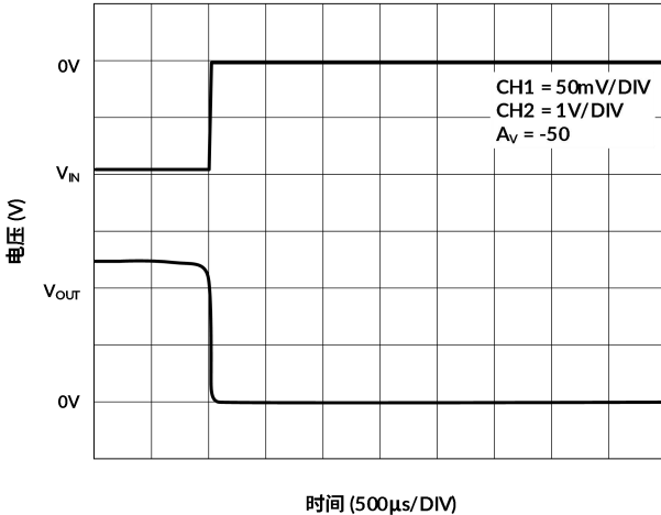
图 32. TLX8547 的负向输入过载恢复
