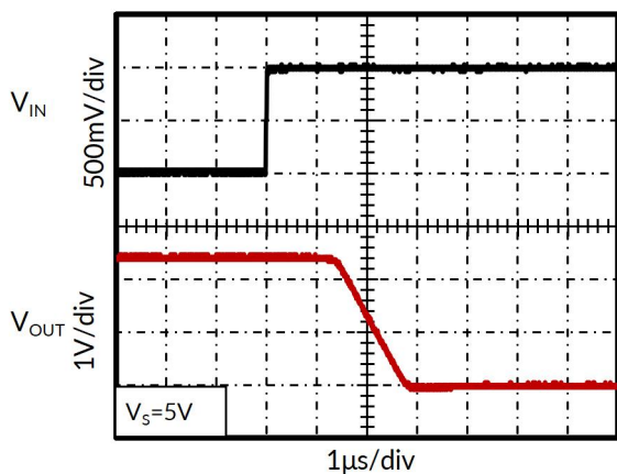
图 21. 反向过载恢复
