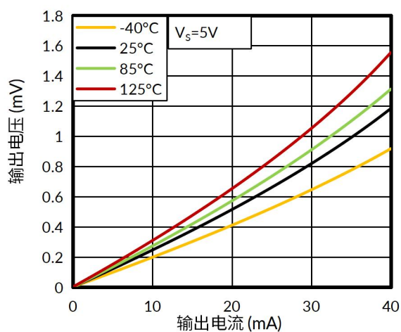
图 4. 输出电压与输出电流的关系（拉电流）
