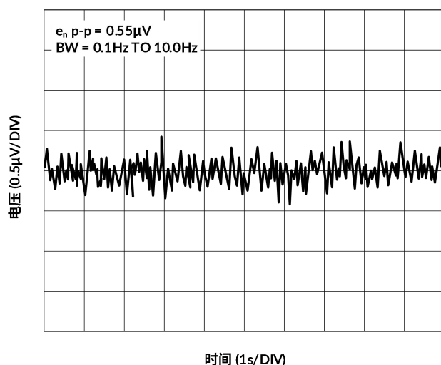
图 23. TLX8547 峰峰值噪声
