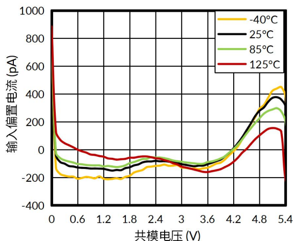
图 6. 输入偏置电流与共模电压的关系
