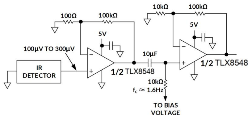
图 35. TLX8548 作为热电堆前置放大器应用方案
