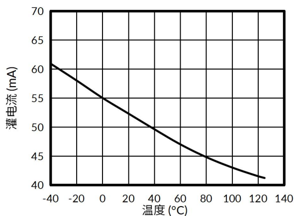
图 10. 灌电流与温度的关系
