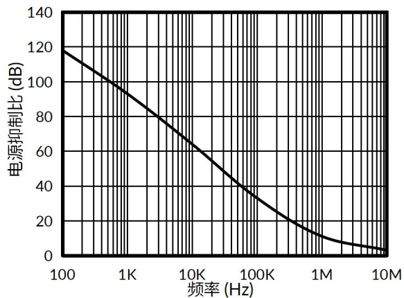
图 5. 电源抑制比与频率的关系
