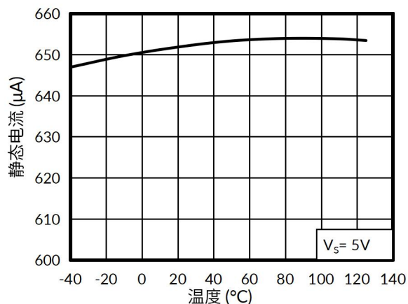
图 7. 静态电流与温度的关系
