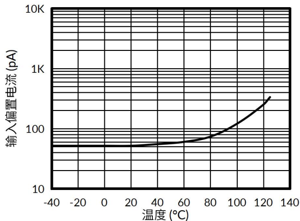
图 4. 输入偏置电流与温度的关系
