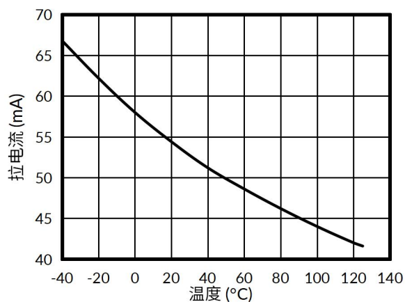
图 9. 拉电流与温度的关系
