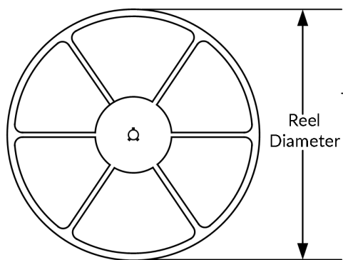
卷盘尺寸
