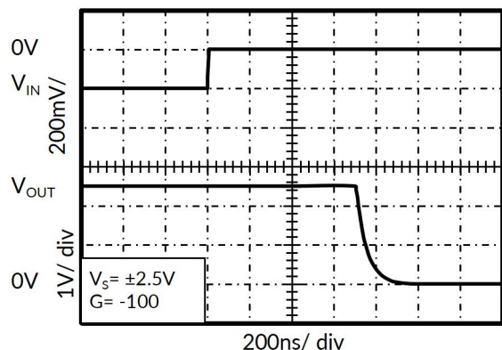
图 13. 正向过载恢复
