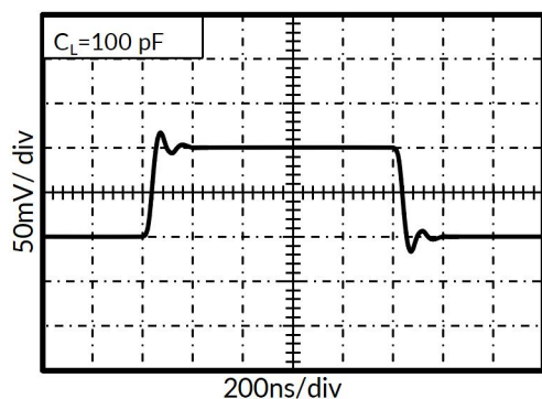
图 11. 小信号阶跃响应
