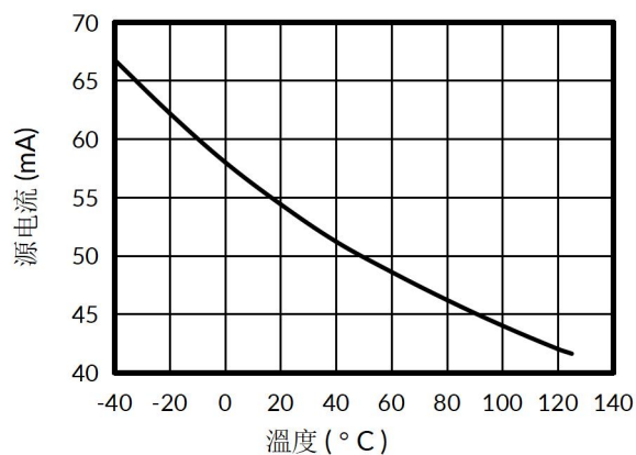
图 9. 源电流与温度
