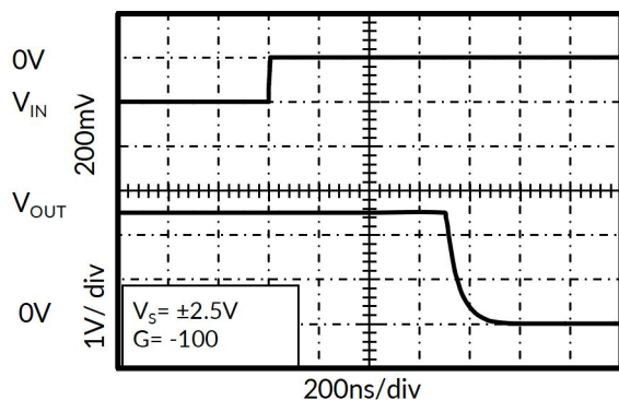
图 13. 正过压恢复
