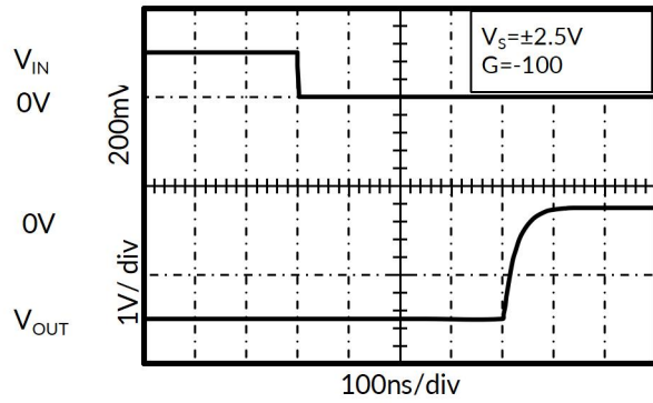
图 14. 反向过载恢复
