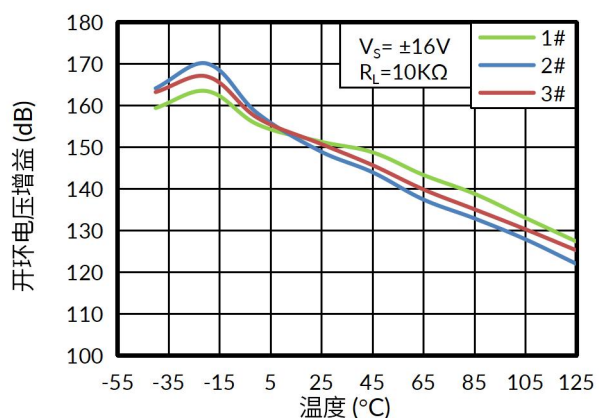
图 10. 开环电压增益与温度的关系
