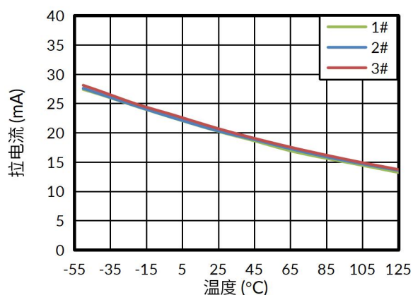
图 9. 拉电流与温度的关系
