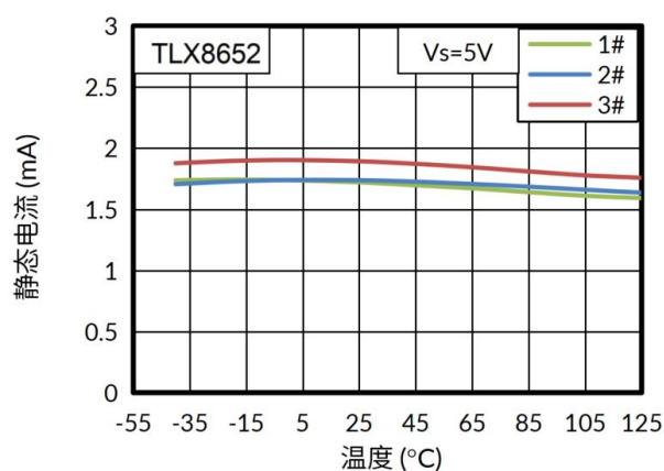
图 4. 静态电流与温度的关系
