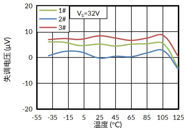
图 2. 失调电压与温度的关系
