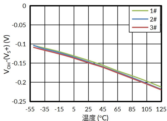
图 7. 输出距轨电压与温度的关系
