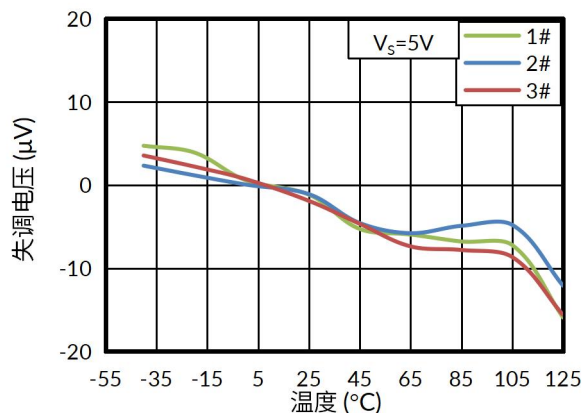
图 1. 失调电压与温度的关系
