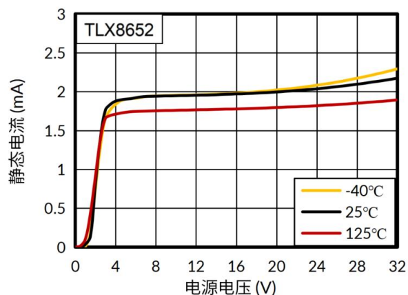
图 3. 静态电流与电源电压的关系
