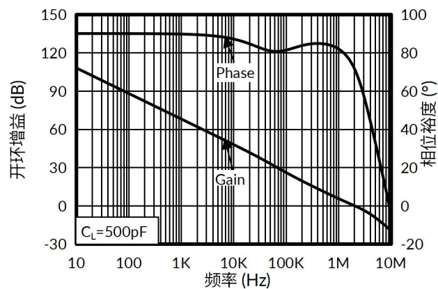
图 13. 开环增益和相位裕度与频率的关系
