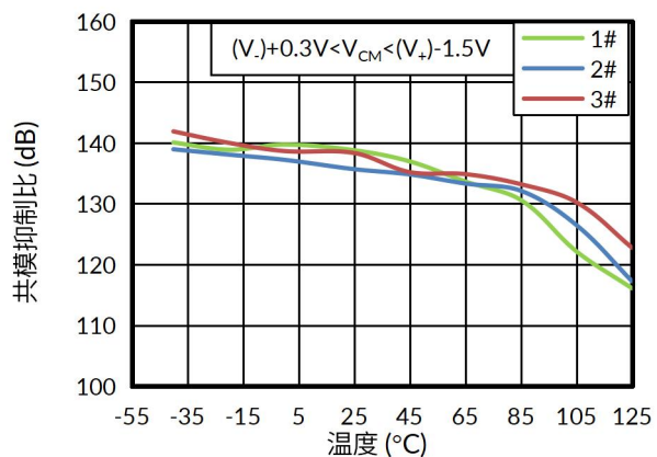
图 12. 共模抑制比与温度的关系
