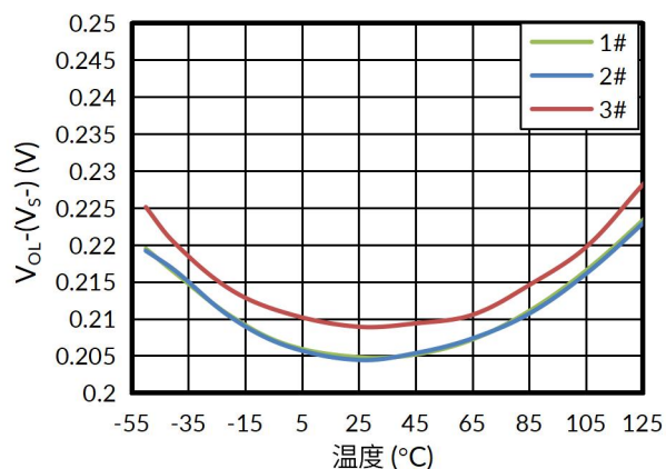
图 8. 输出距轨电压与温度的关系
