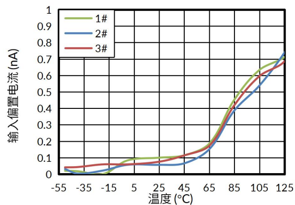
图 6. 输入偏置电流与温度的关系
