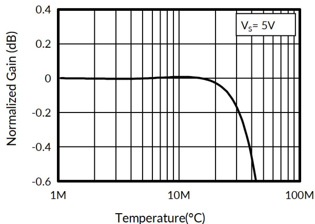
图 6. 交流响应
