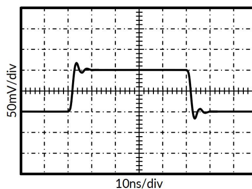
图 10. 小信号阶跃响应
