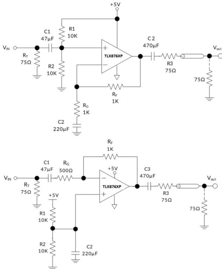
图 13. 5V 单电源同相和反相视频线路驱动器
