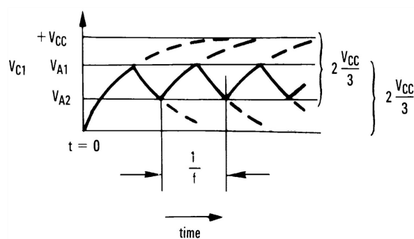
图 8. 方波振荡器
