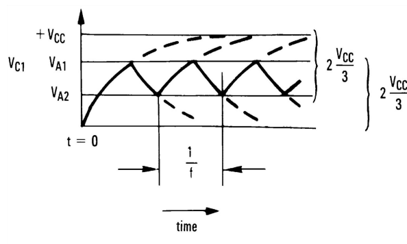
图 8. 方波振荡器
