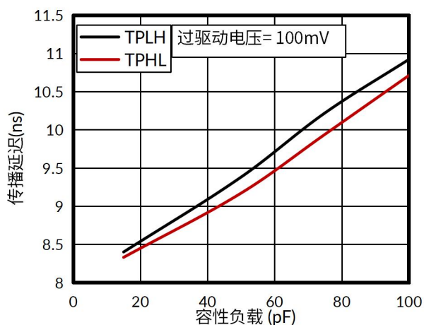
图 6. 传播延迟与容性负载的关系
