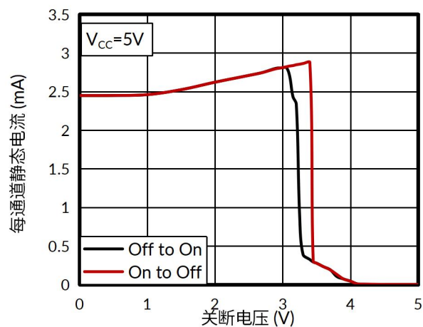
图 11. 静态电流与关断电压的关系
