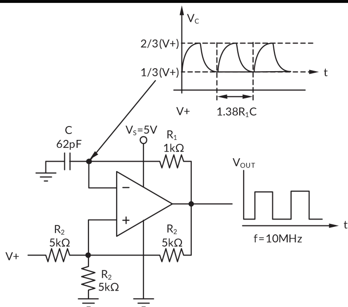
图 17. 弛张振荡器
