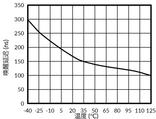
图 4. 唤醒延迟与温度的关系
