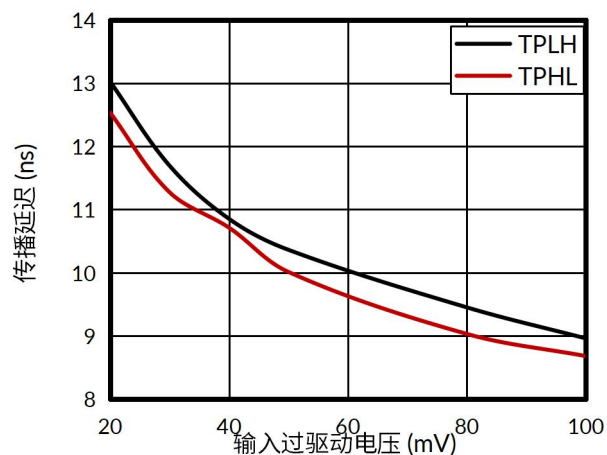
图 7. 传播延迟与输入过驱动电压的关系
