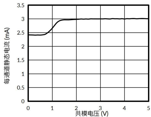
图 13. 静态电流与共模电压的关系
