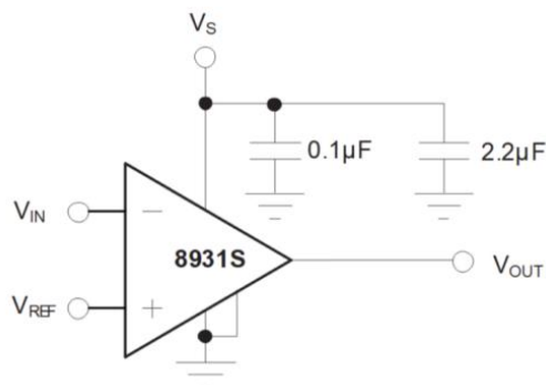
图 15. TLX8931S 基本连接
