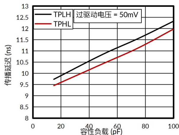
图 5. 传播延迟与容性负载的关系
