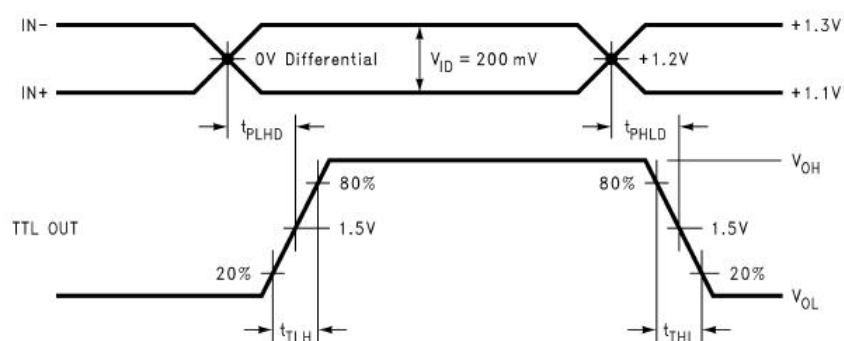
图 4 传输延时和转换时间示意图
