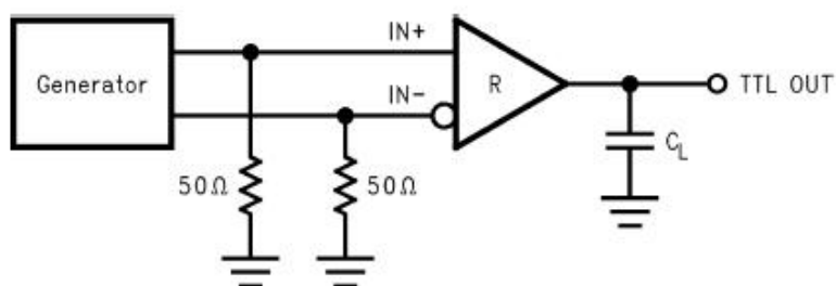
图 3 瞬态特性测试电路框图
