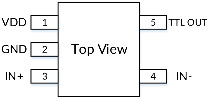
图 2. TLX90LV012 引脚配置
