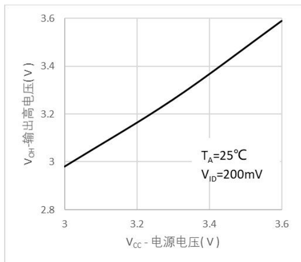
图 2. 输出高电压 vs 电源电压
