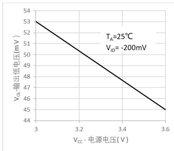
图 3. 输出低电压 vs 电源电压
