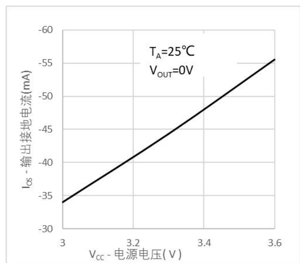
图 4. 输出接地电流 vs 电源电压
