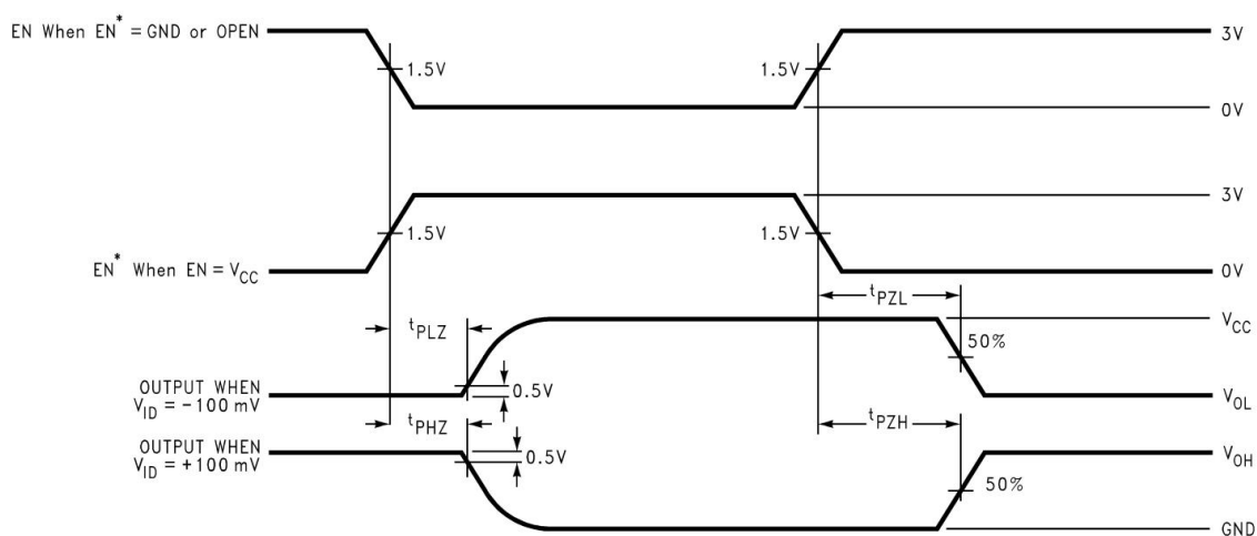
图 9. 接收器高阻态延时波形图
