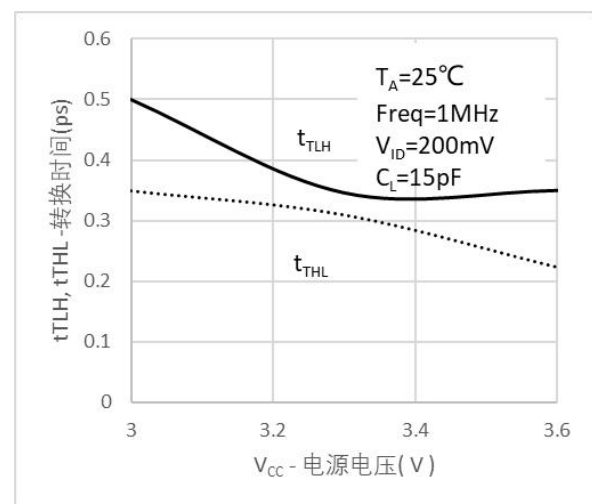
图 5. 转换时间 vs 电源电压
