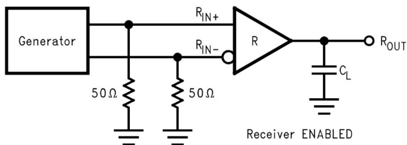
图 6. 传输延时和转换时间测试电路框图
