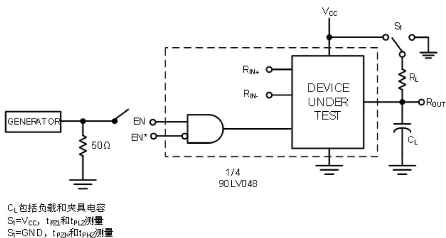
图 8. 接收器高阻态延时测试电路框图
