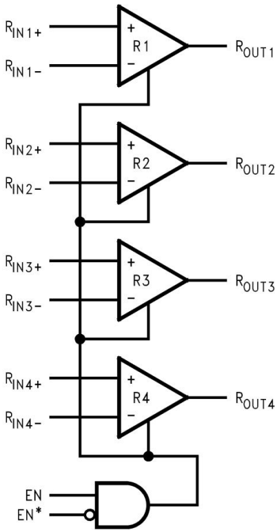
图1. TLX90LV048功能框图
