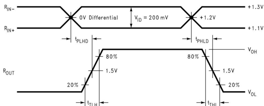
图 7. 传输延时和转换时间波形图
