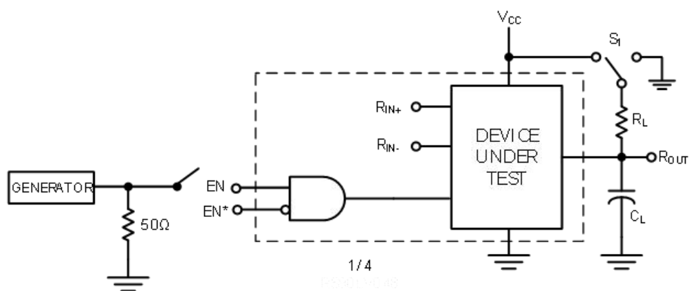
图 3. 传输延时和转换时间示意图
