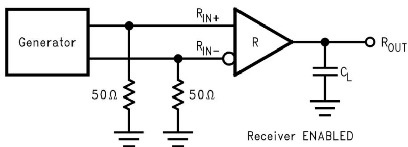
图 2. 瞬态特性测试电路框图
