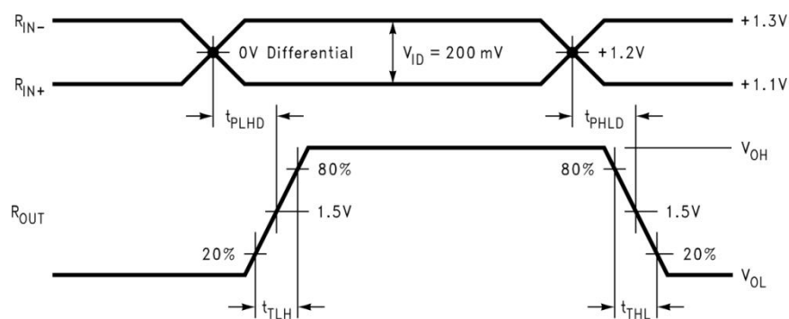
图 3. 传输延时和转换时间示意图
