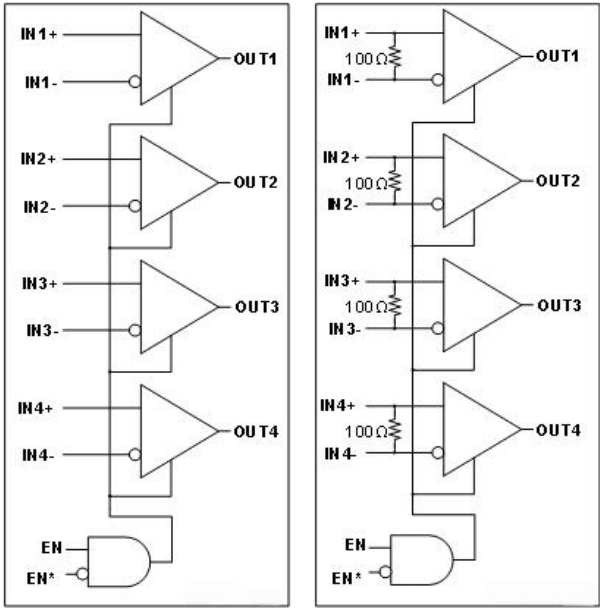
图 1. 功能框图
