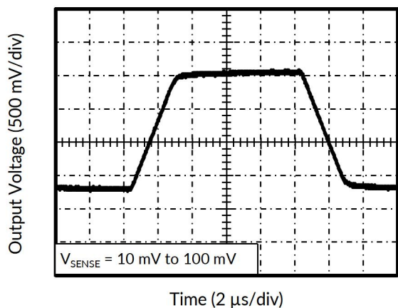
图 13. 阶跃响应
