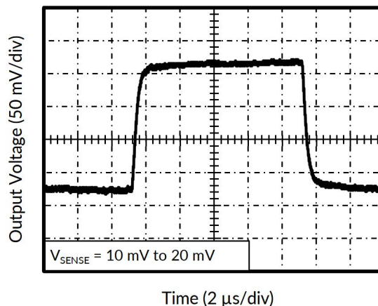
图 12. 阶跃响应
