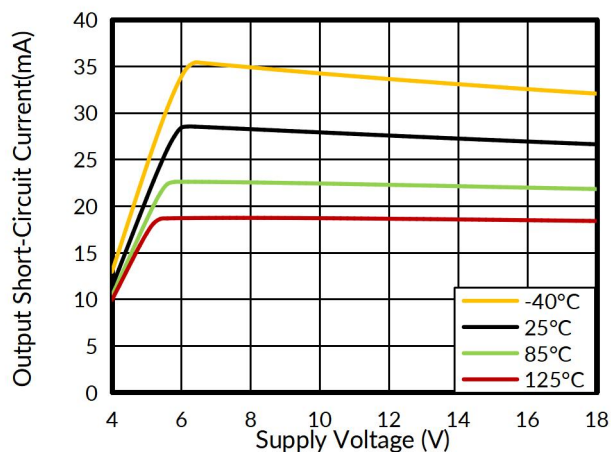
图 11. 输出短路电流与电源电压
