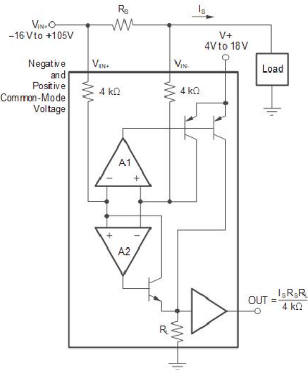
简化示意图
