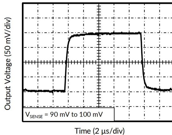
图 14. 阶跃响应
