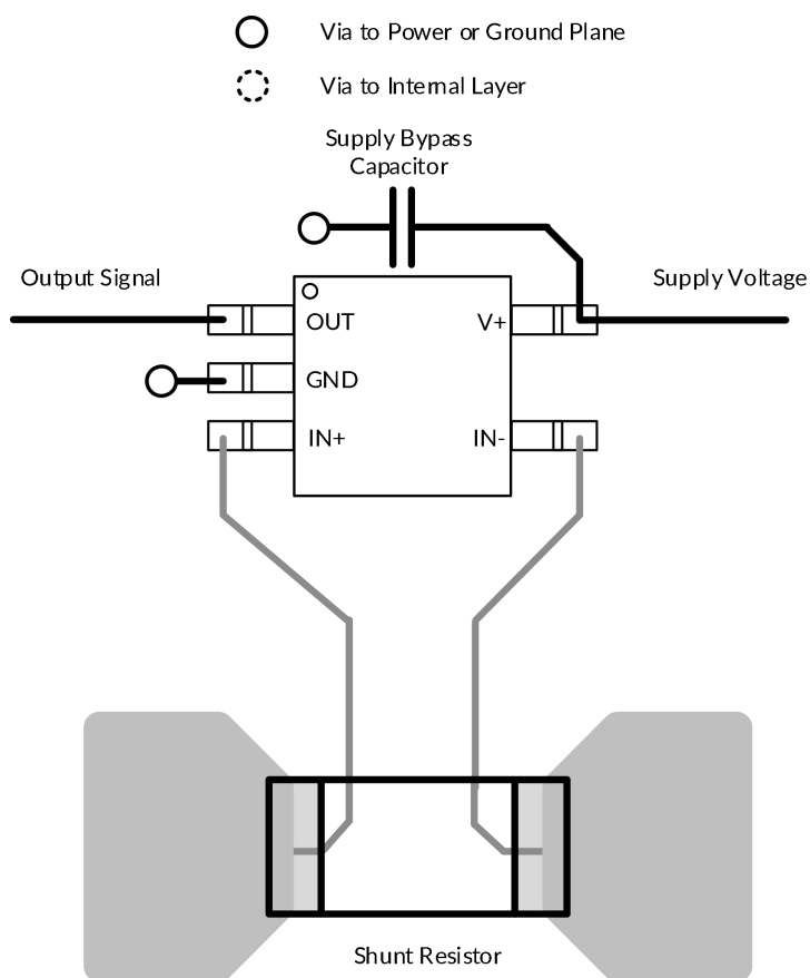
图 24. 推荐布局
