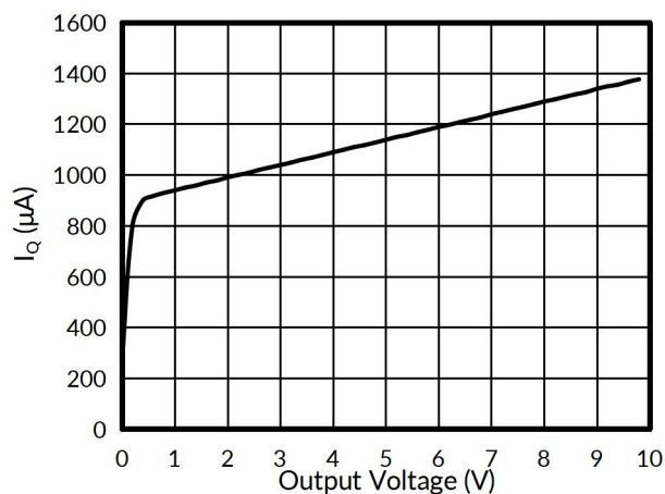
图 7. 静态电流与输出电压的关系
