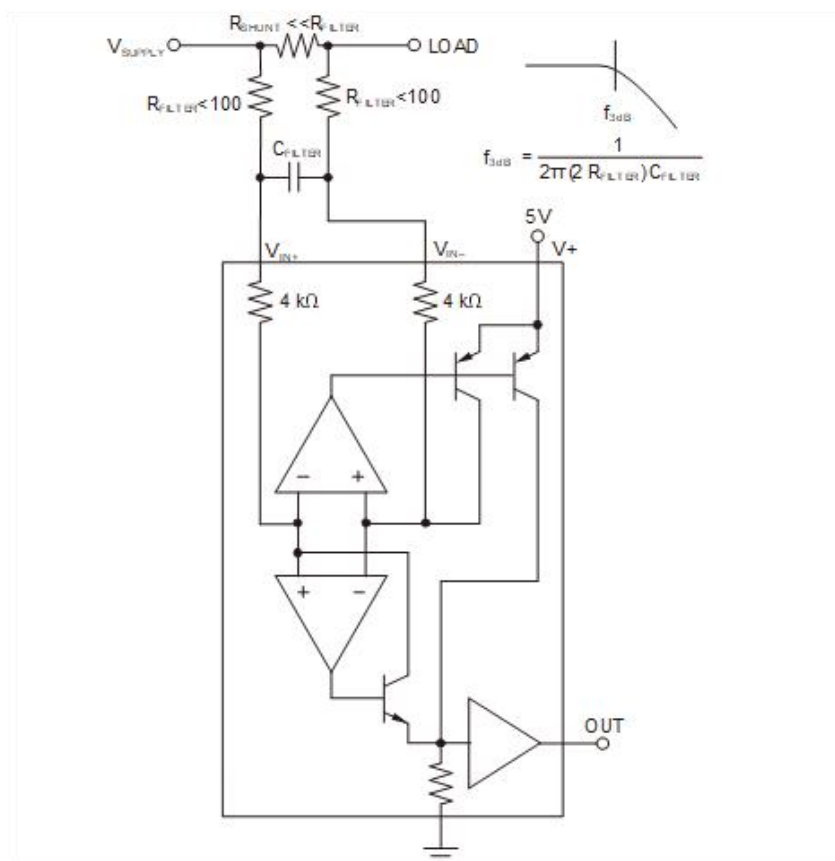
图 20. 输入滤波器
