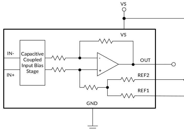
图 18. V_S 参考输出
