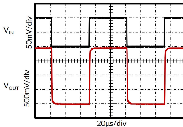
图 10. 大单步响应
