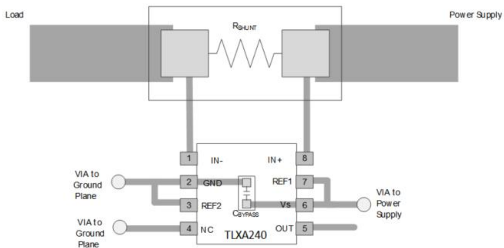
图 27. 推荐的 SOP 封装布局
