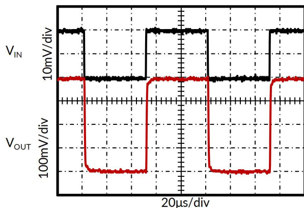
图 11. 小-单步响应
