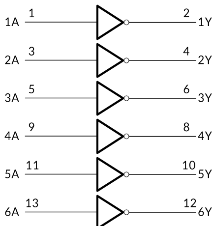
功能框图
